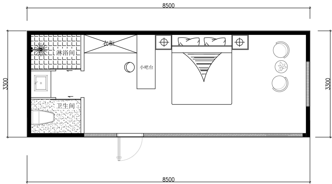
平面布置图
